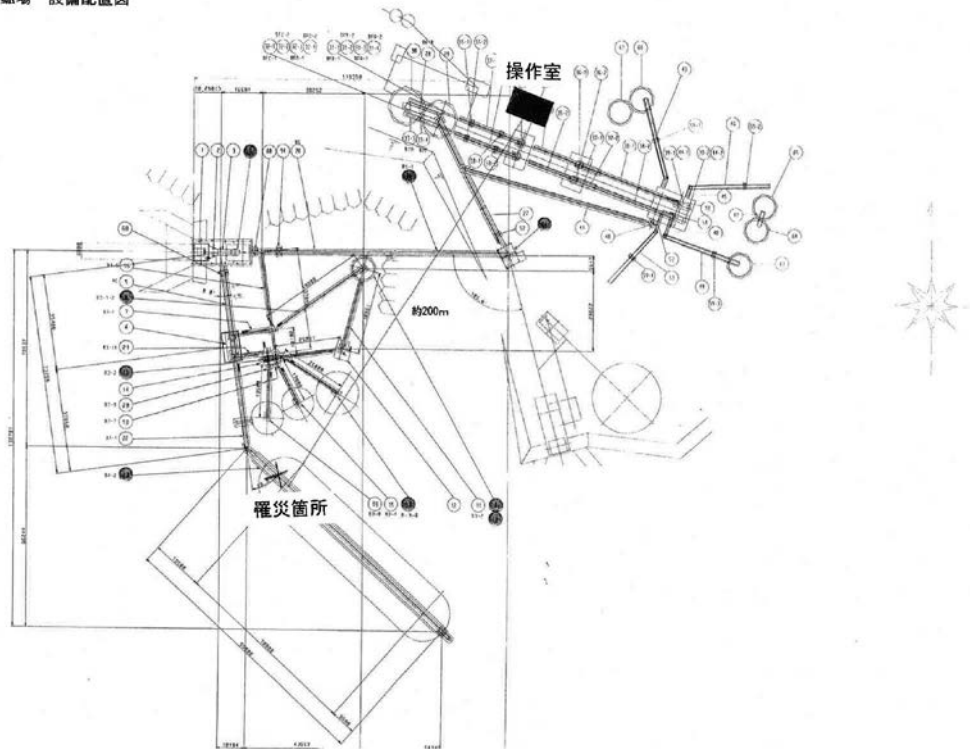
選鉱場 設備配置図
