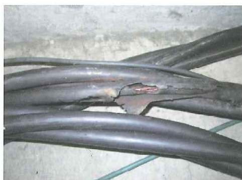
写真1 絶縁破壊したケーブル
